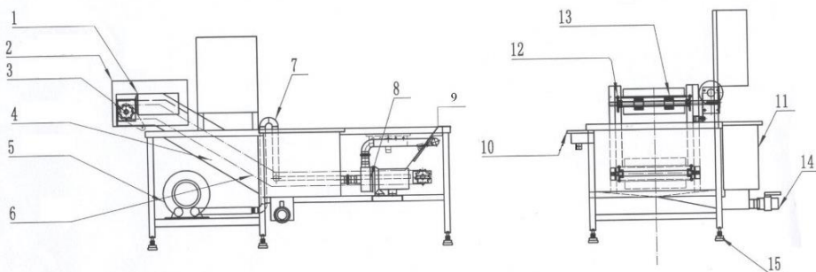
Рис 1. Основные элементы оборудования
